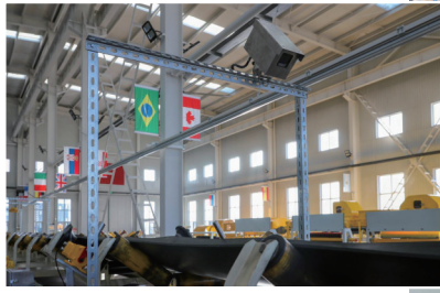
图为带式输送机视觉AI智能型自动纠偏系统样机。
